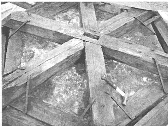
Belki podwaliny podstawy kopuły nad kaplicą
